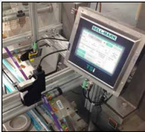
Montiert an einem Continuous Motion Flow Wrapper
